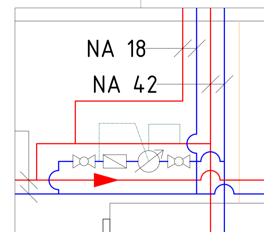
Hőmennyiségmérő beépítése részletraaj
